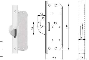
Reteszes (D-dual) másodzár:
