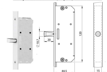
Kampós reteszes (H-hook) mellékzár:
