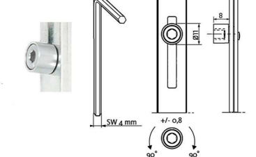
Csapos reteszes (P-pin) mellékzár:
