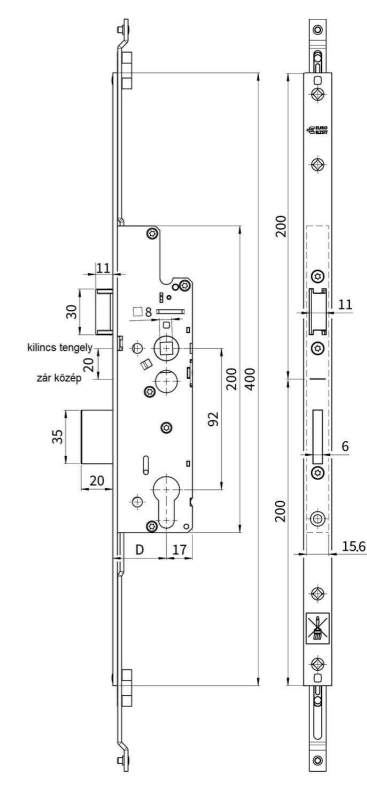
Hengeres (R-roller) görög:
